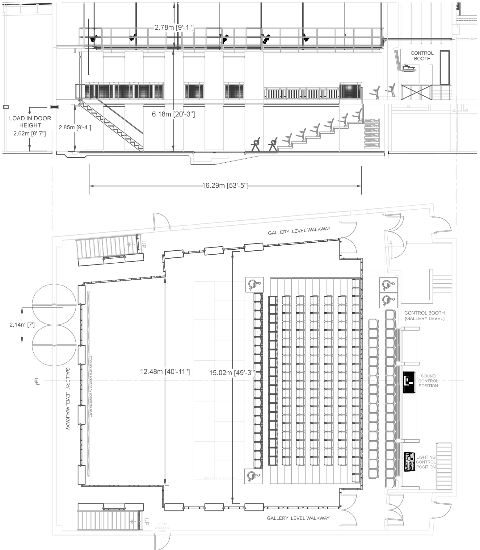
Studio du Théâtre Centrepointe Studio Theatre Plan & Section View, Voir plan et coupe Configuration standard configuration
